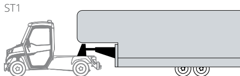
ST1 Version für das Ziehen eines Sattelauflegers mit automatischer Anhängerkupplung DIN Ø40
