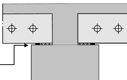
Oplegdetail tussensteunpunt
