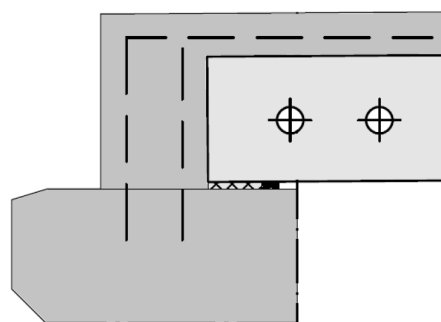
Oplegdetail landhoofd
