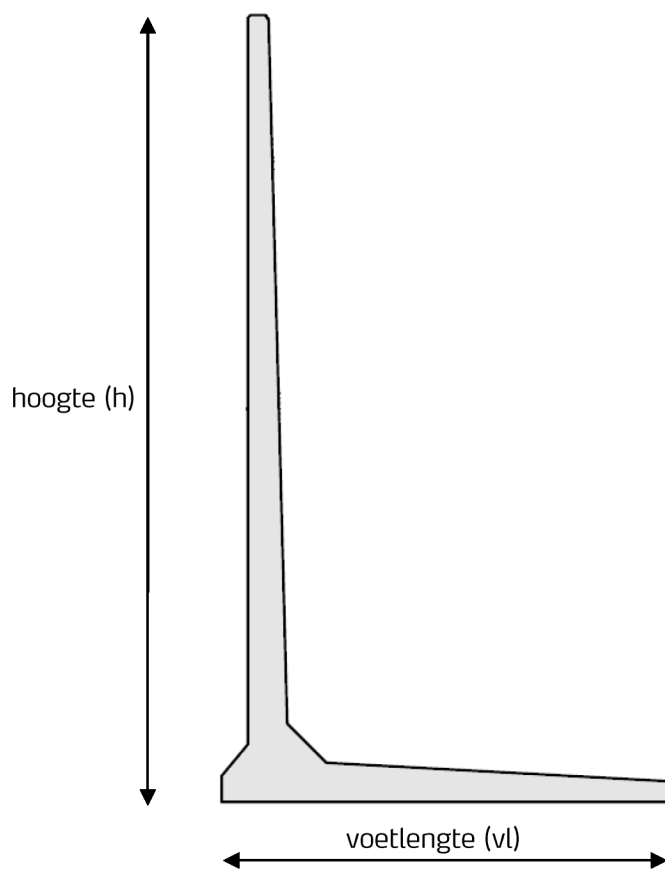
Voorbeeld dwarsdoorsnede
