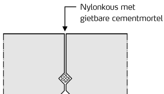
Voegdetail
