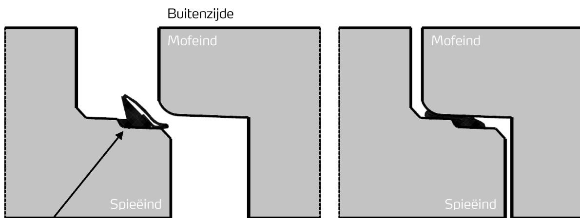
Voegdetail R1-rubberring duiker
