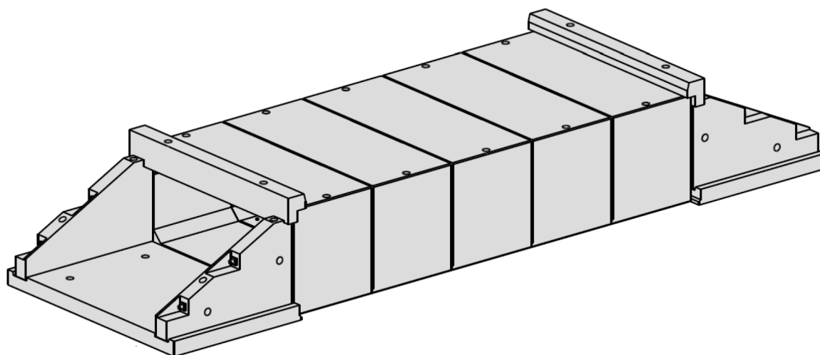
3D Aanzicht van de duiker met taludbeëindigingen
