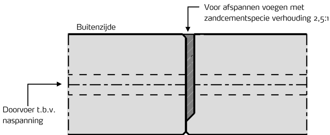
Voegdetail
