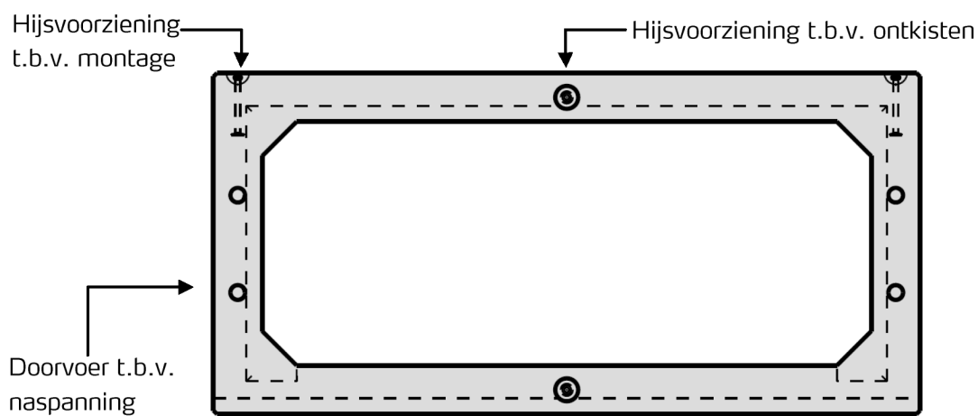
Aanzicht duikerelement
