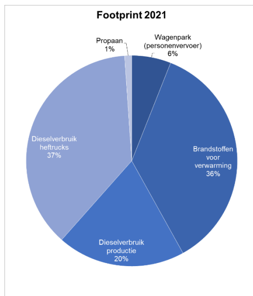
Figuur 1: CO 2 -footprint van De Hamer
