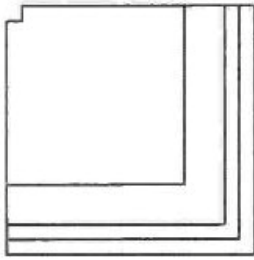
Abb. 1. Innere Ecklösung 90° 0,75 m bis 3,00 m hoch
