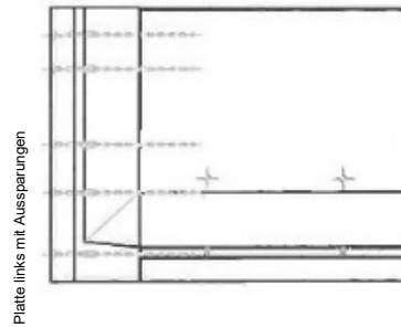
Abb. 4 Äußere variable Ecklösung
