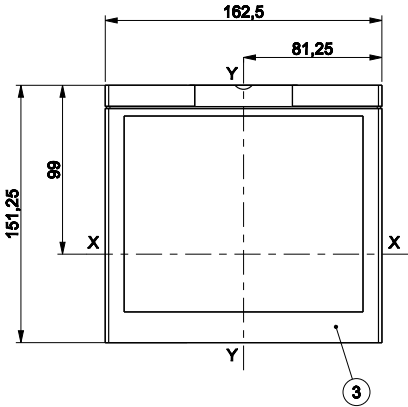
Flange
