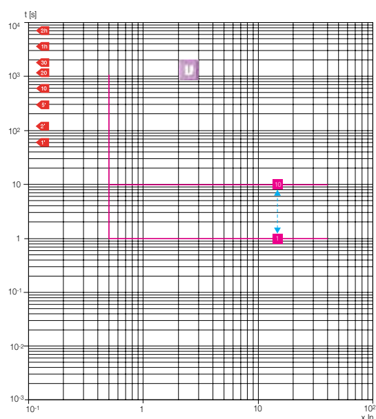
XT2 Ekip M Touch LRIU U function
