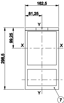
Flange
