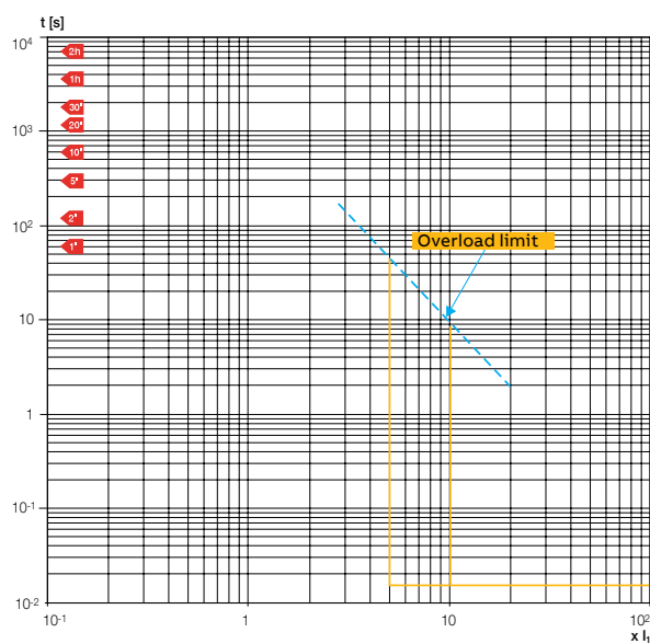
XT4 200 MA I_n=10\ldots200\text{A}
