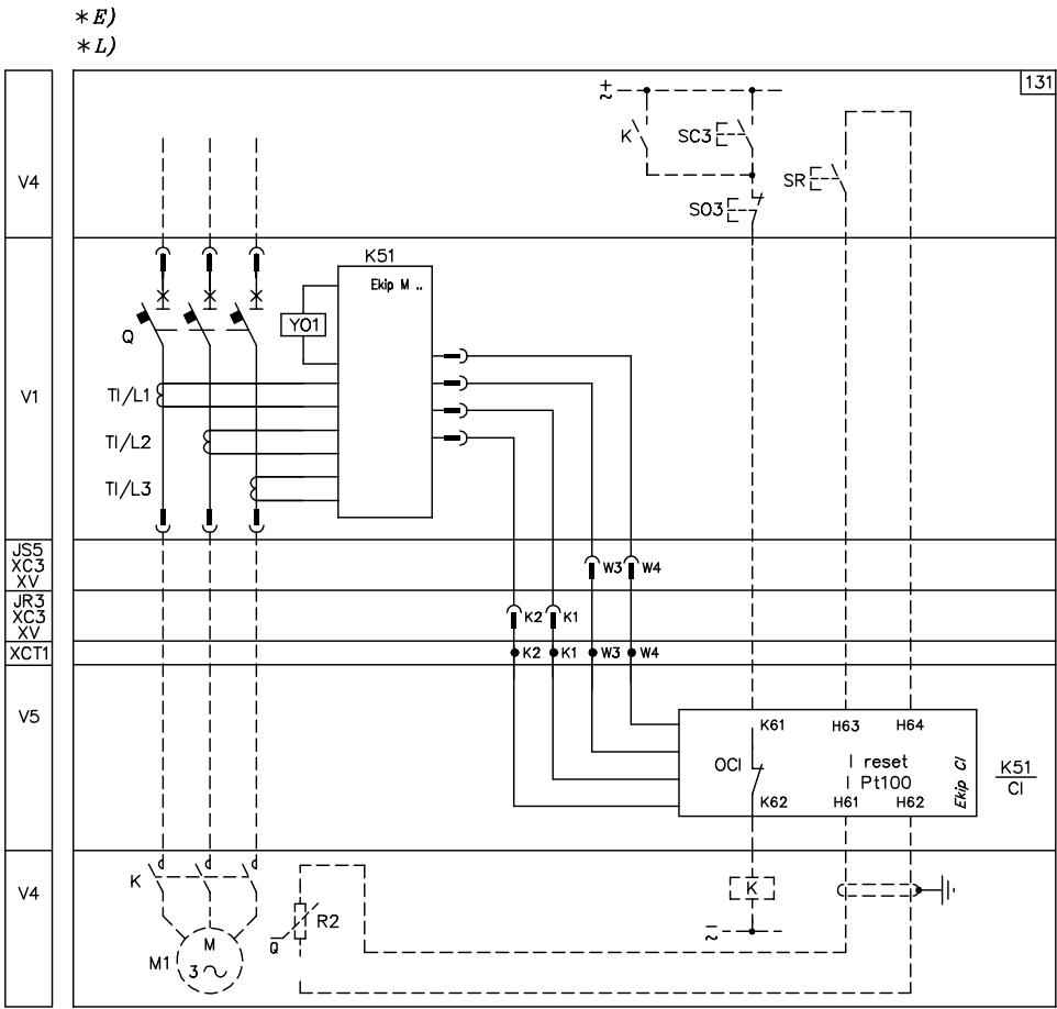
131) Motor starting module Ekip CI
