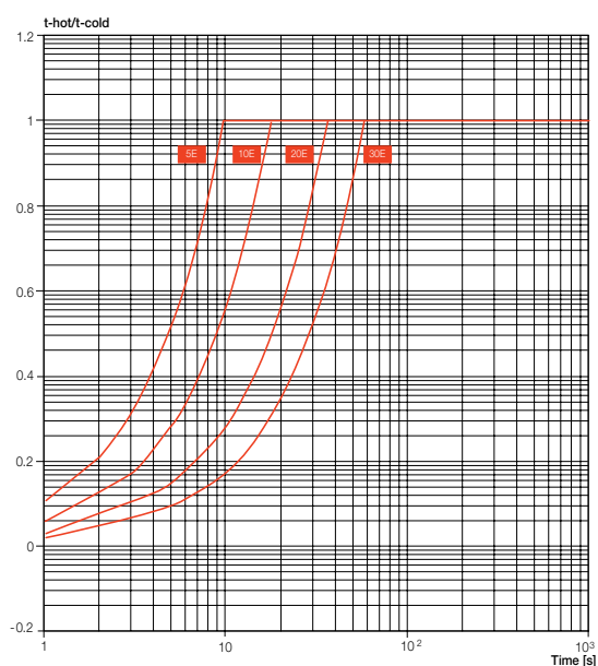
XT5 Ekip M Touch LRIU (hot trip)
