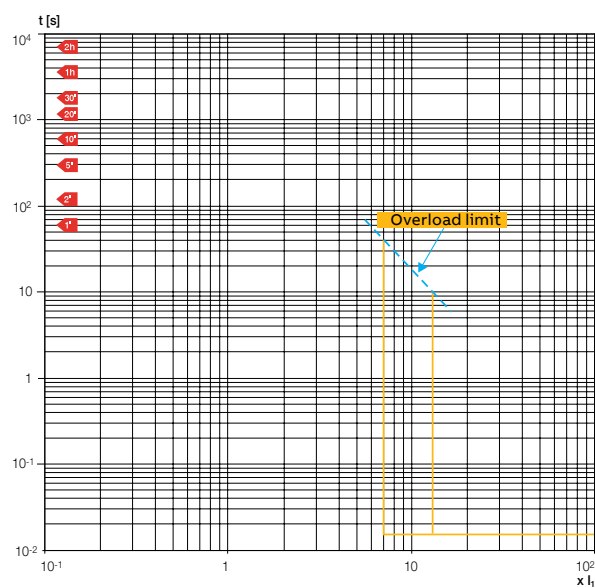
XT5 400-630 MA I_n=320\ldots500\text{A}
