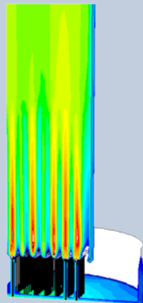
Resultados sem vento CFD – Temperatura na Linha de Centro (F)
