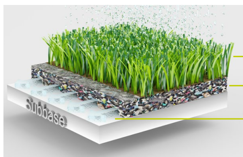
Kunstrasensystem mit ProPlay®-Sport Elastikschicht- und Entwässerungsauflage
