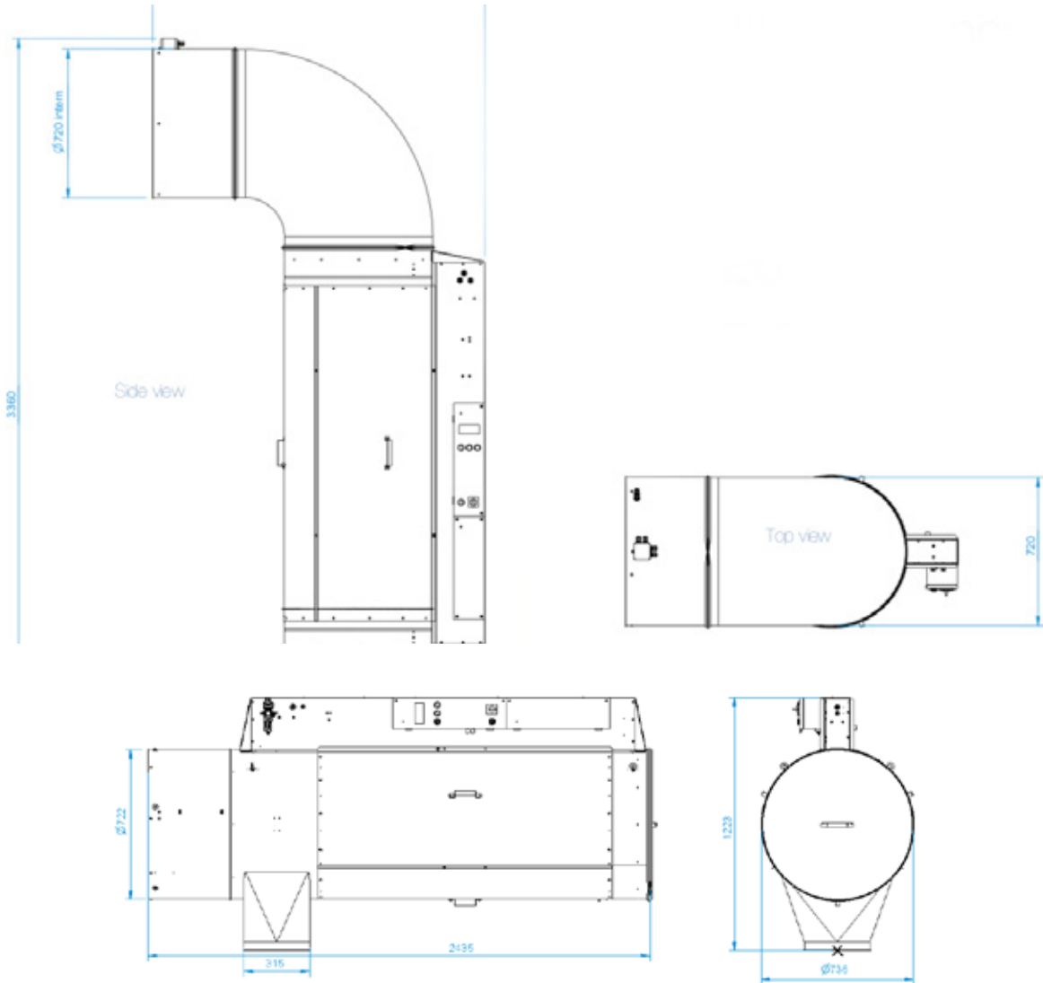
PARTIKKELIT
