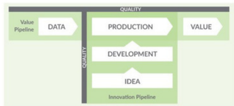
DataOps
