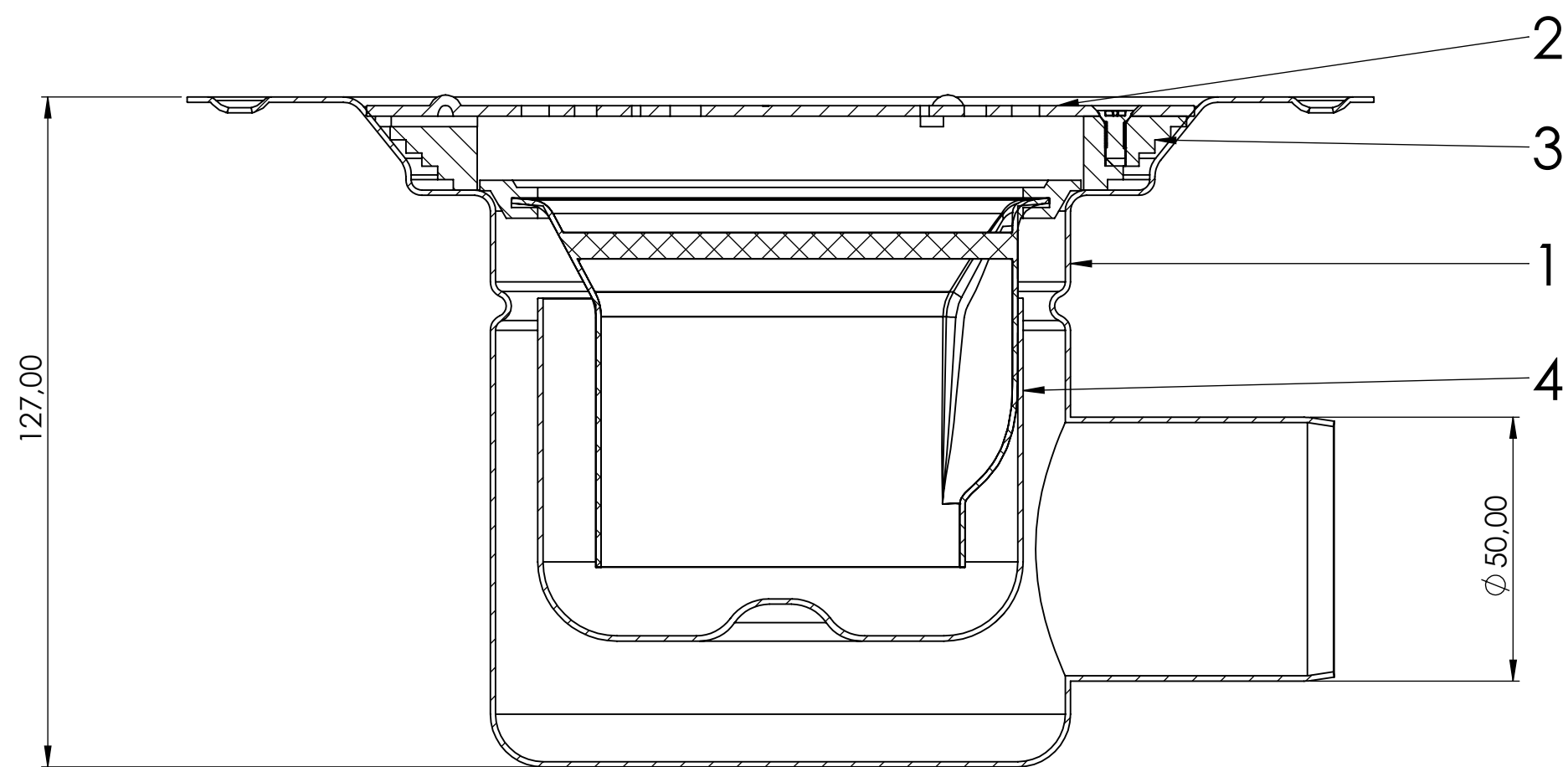
SECTION A-A
