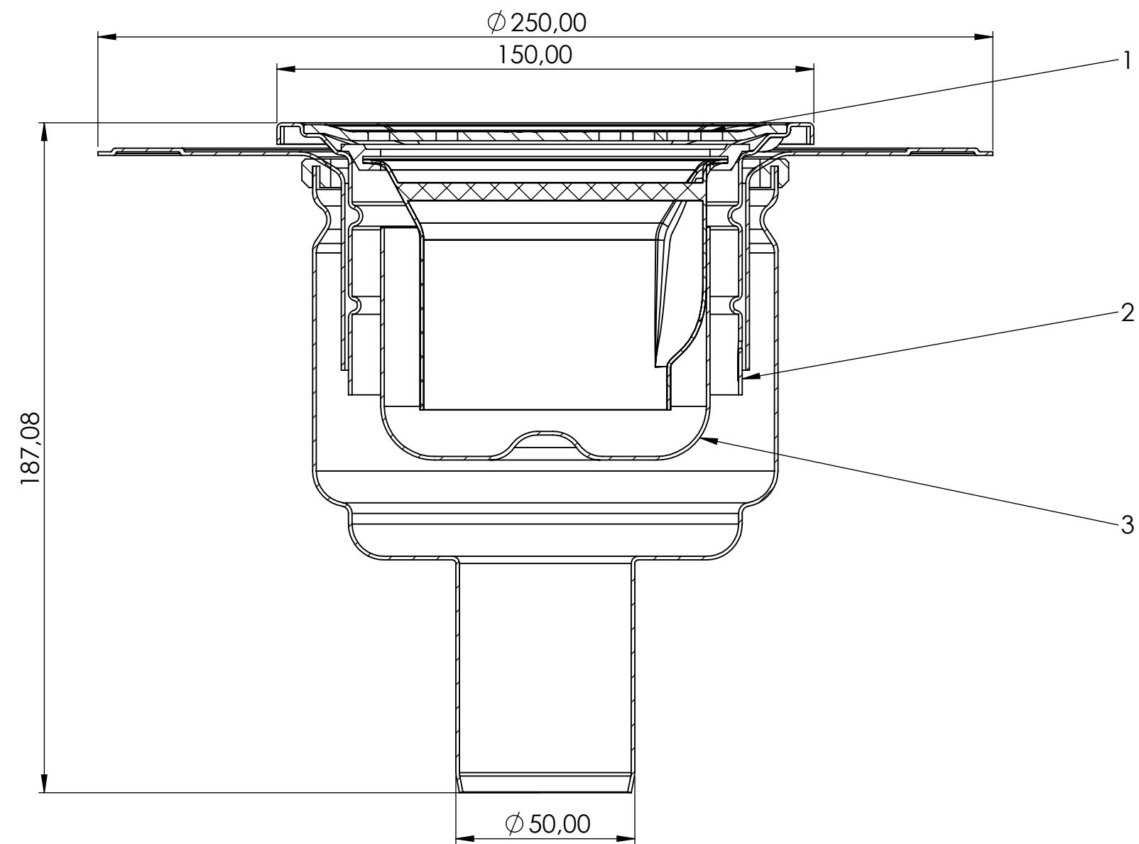
SECTION A-A SCALE 1 : 1.5
