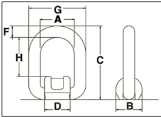
S-265 Weld-On Pivot Link
