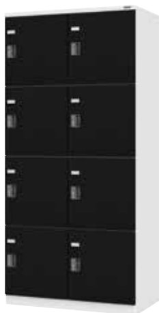
TH2-4C (2列4段 8人用) H1900×W900×D510 横中仕切板溶接固定、扉(補強付)、 プラスチック名札差 付
